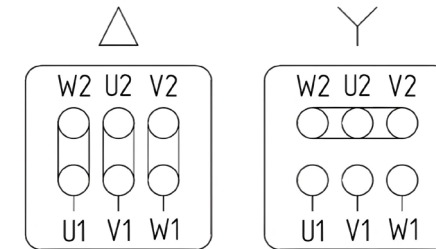
Рисунок – 5. Схема соединения обмоток электродвигателя
