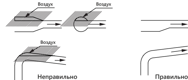
Рисунок – 4. Правильный монтаж трубопроводов
