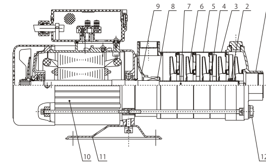
Рисунок – 2. Конструкция насоса серии ВНР
